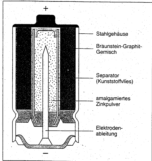
Schnitt durch eine Alkali-Mangan-Batterie
