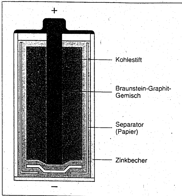
Schnitt durch ein LECLANCHE-Element
